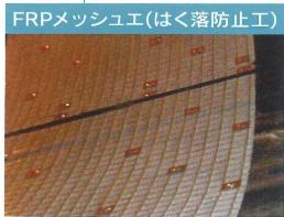
FRPメッシュ工(はく落防止工)
